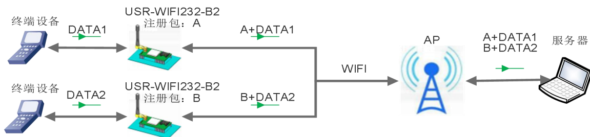
图 35 数据携带注册包框图
