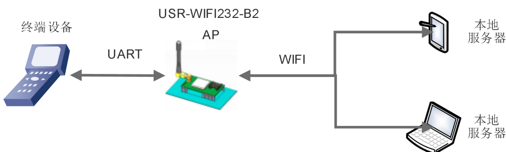
图 12 USR-WIFI232-B2 自组网 1
