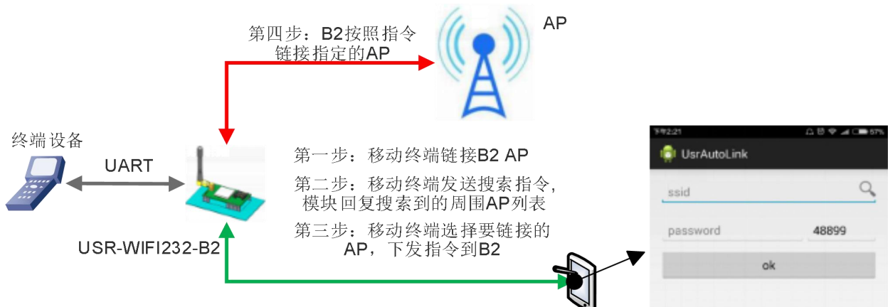
图 39 usr-link 框图
