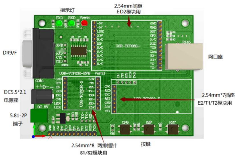
图 5 USR-TCP232-EVB
