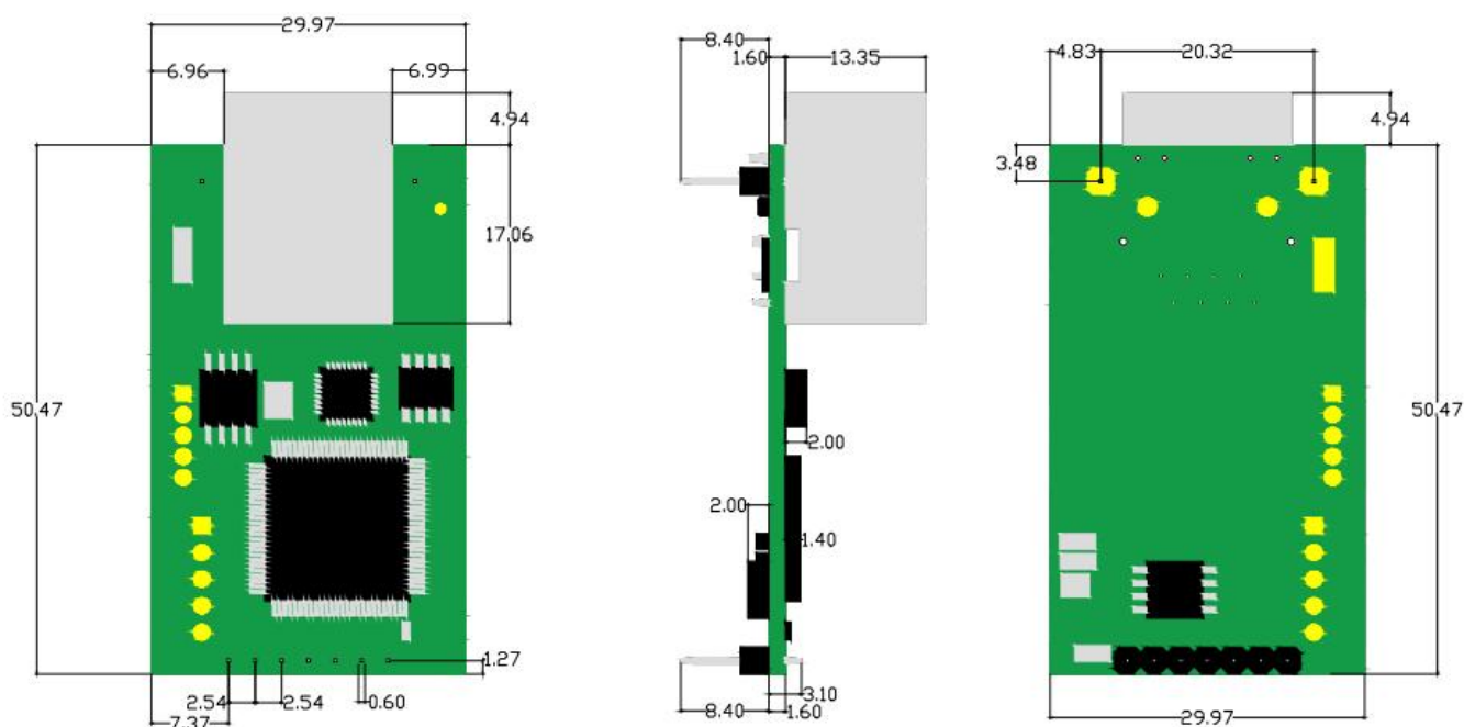
图 1 USR-TCP232-E2 尺寸示意图
