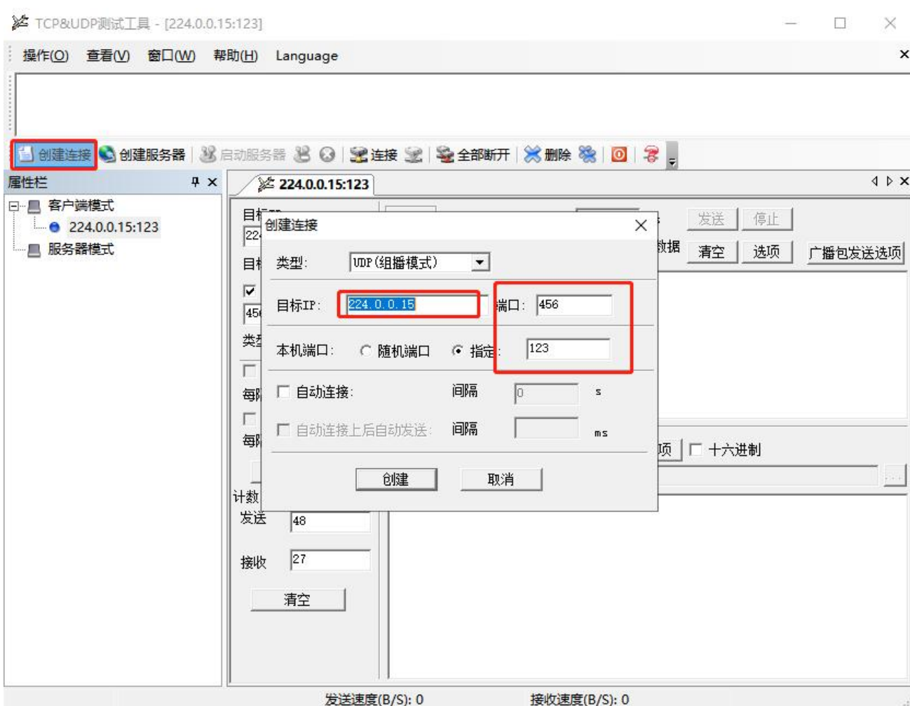
图 33 UDP 组播连接
