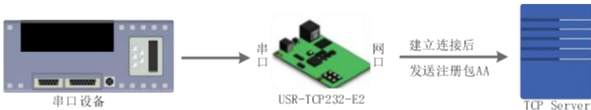
图 56 建立连接发送注册包
