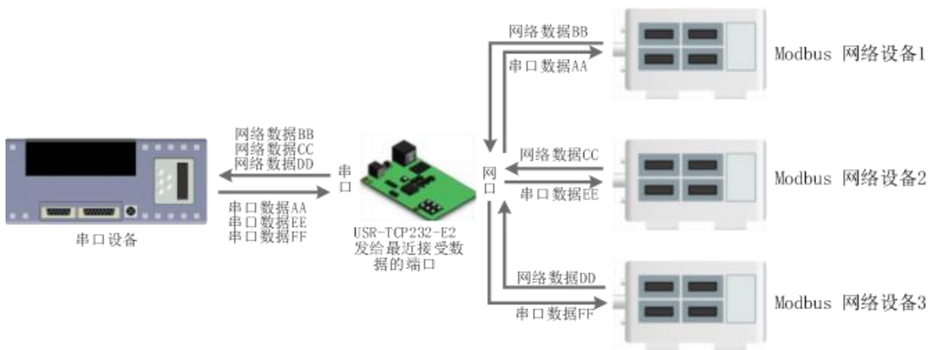
图 67 Modbus TCP
