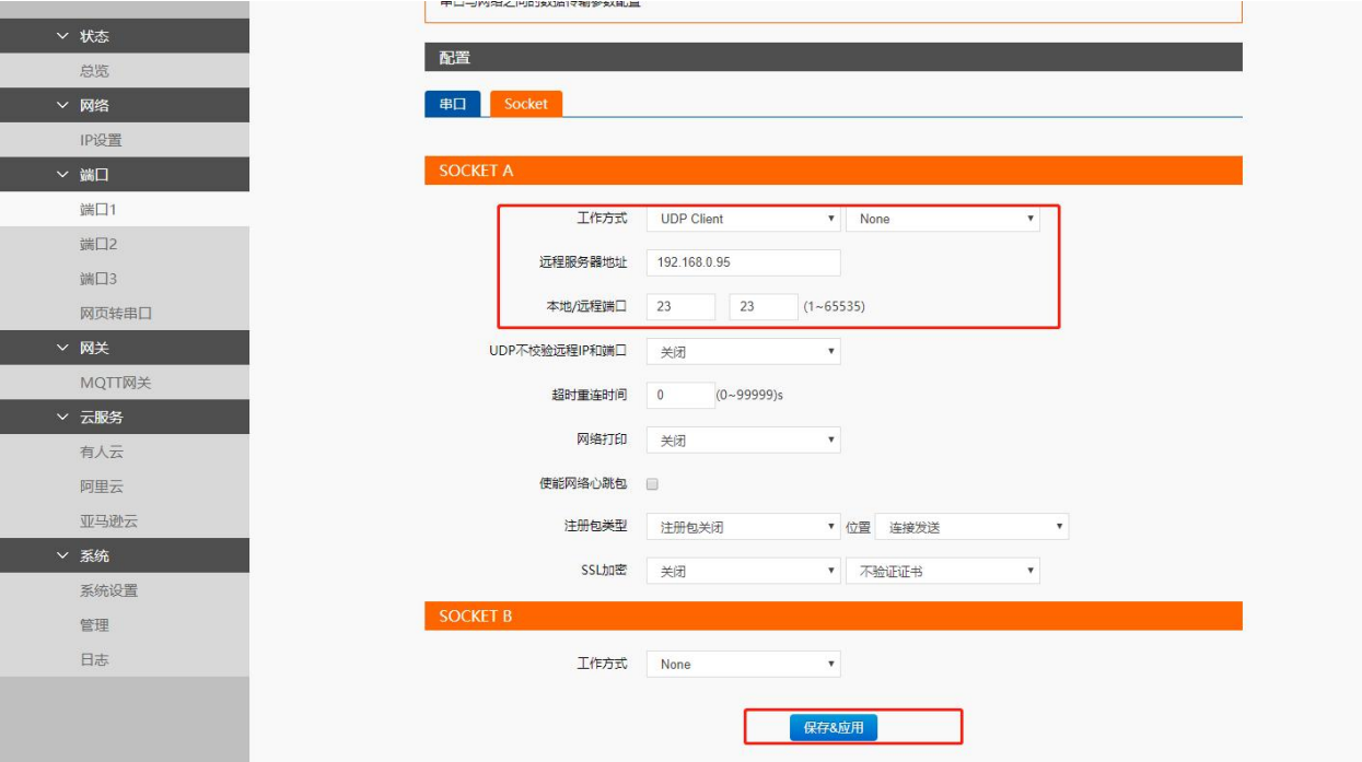
图 30 UDP Client 网页设置
