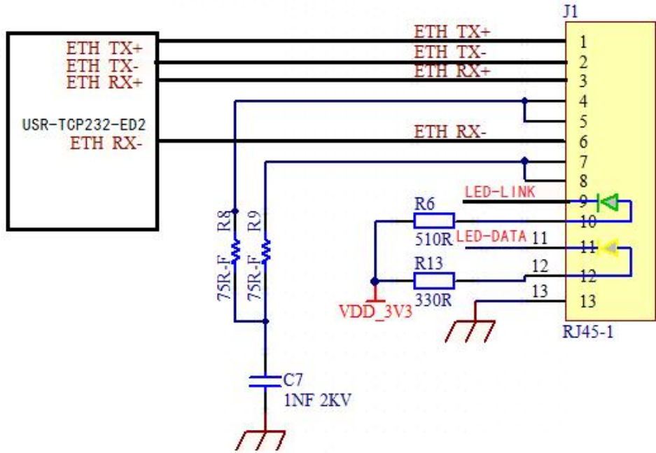
图 12 USR-TCP232-ED2 模块网口的应用
