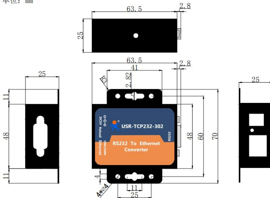
图 1. USR-TCP232-302 尺寸图
