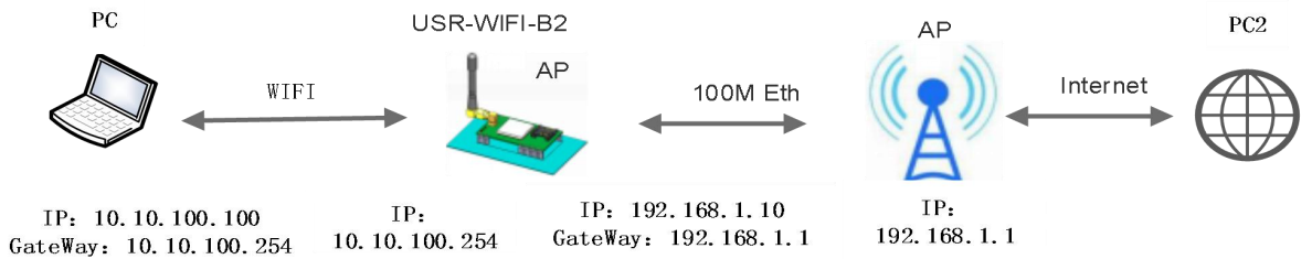
图 18 有线加无线组网应用（AP WAN）
