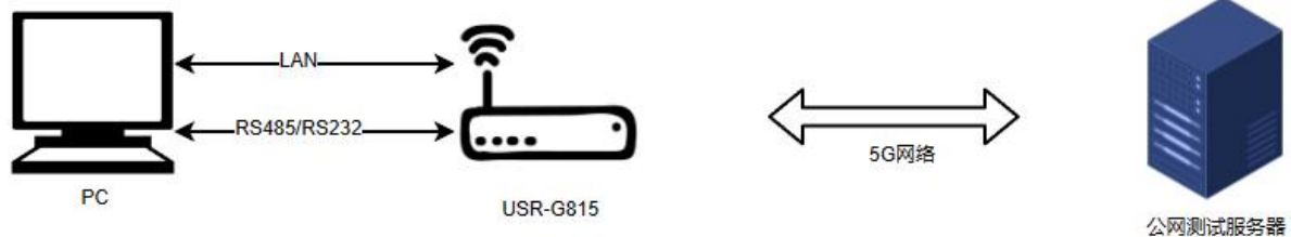
图 44 串口透传拓扑
