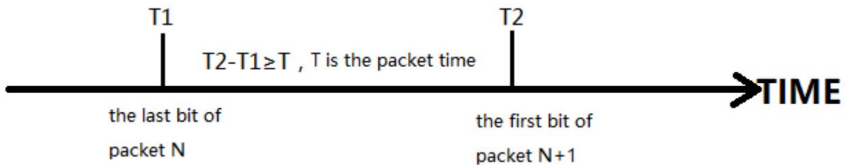
图 17 时间触发模式
