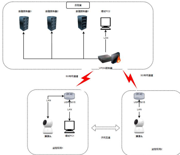
图 38 专网卡实现远程监控拓扑
