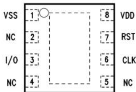
图 12 C2x2eSIM 芯片管脚示意 (TOP VIEW)
