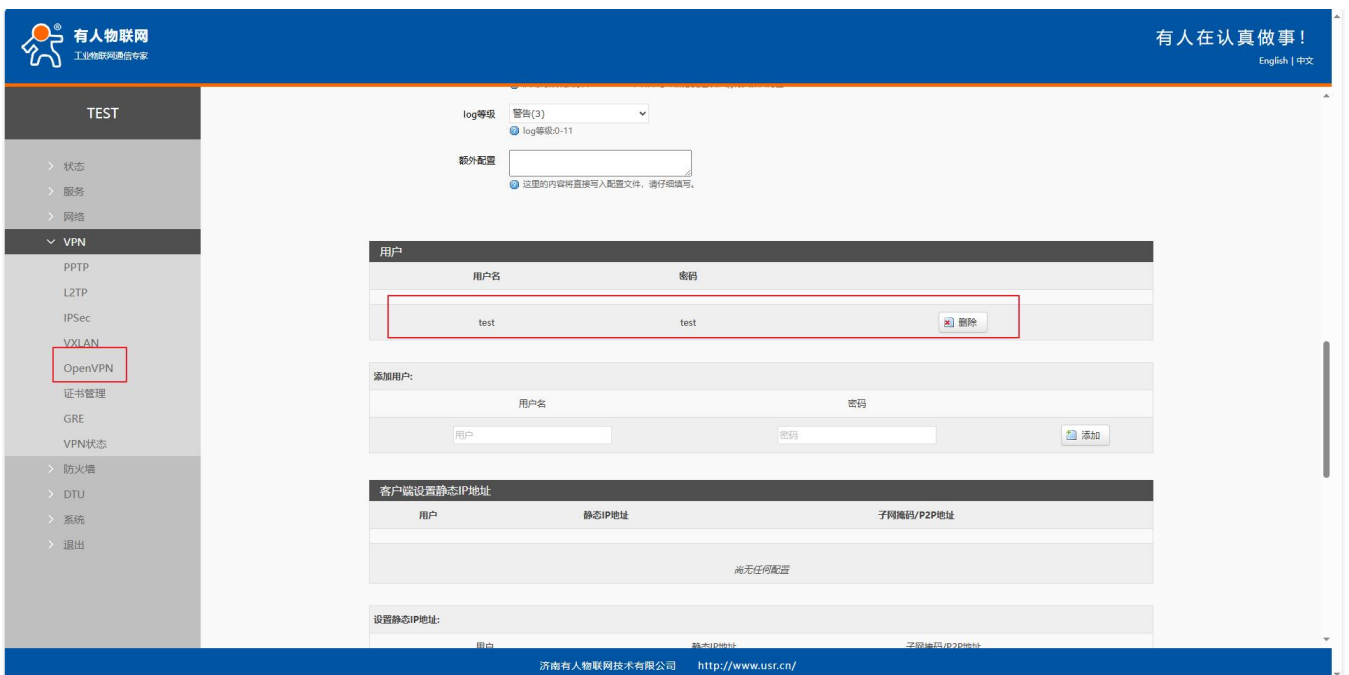
图 65 Openvpn 配置 2
