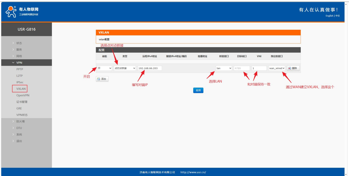
图 53 路由器 1 配置
