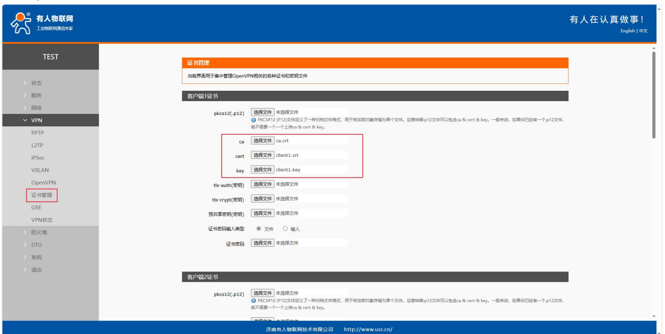
图 78 路由器 2 配置 3
