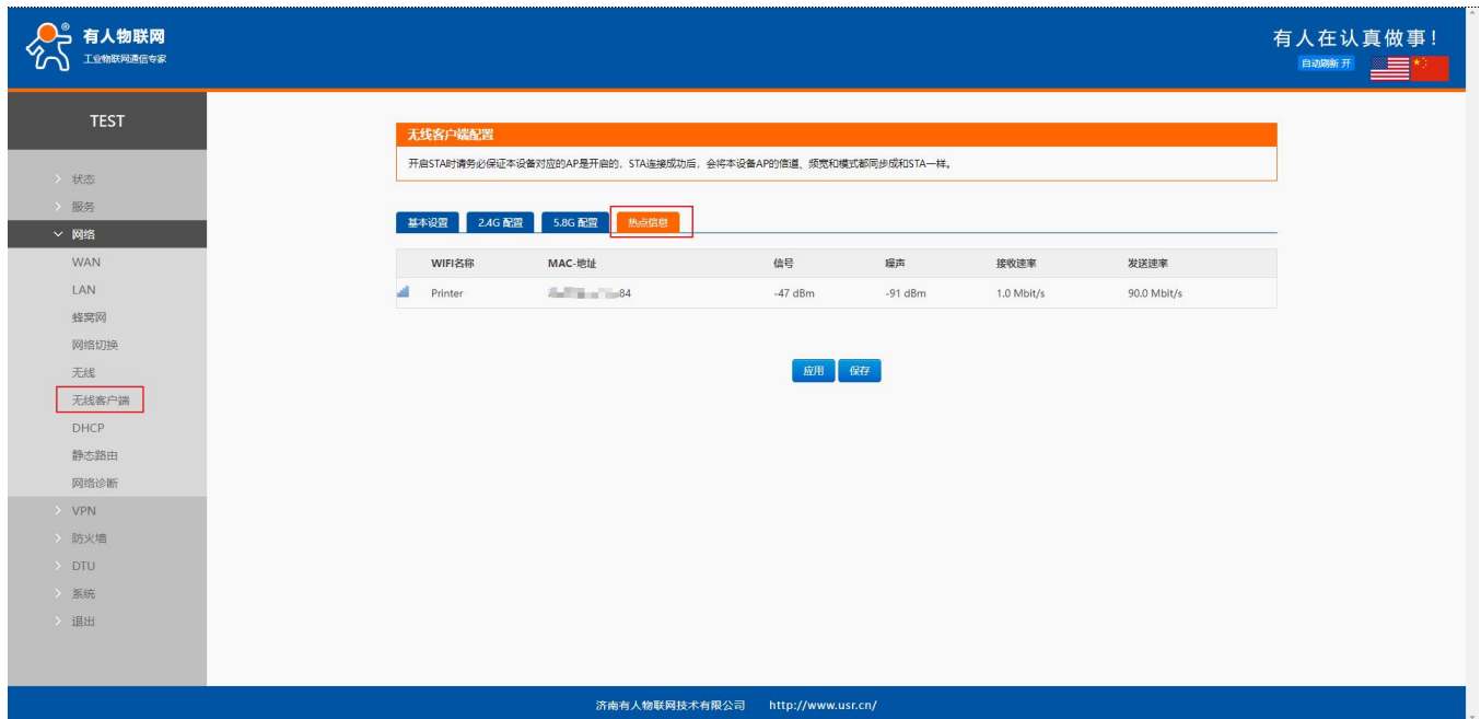
图 36 热点信息
