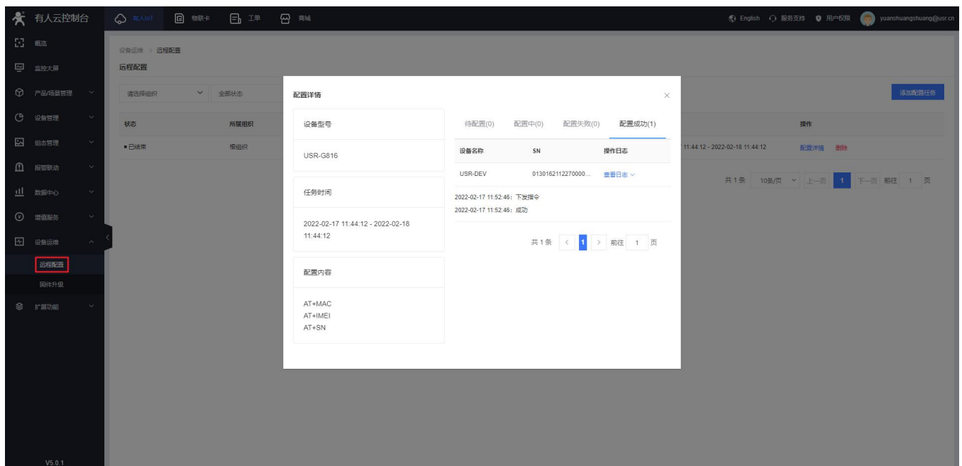
图 118 远程配置（四）
