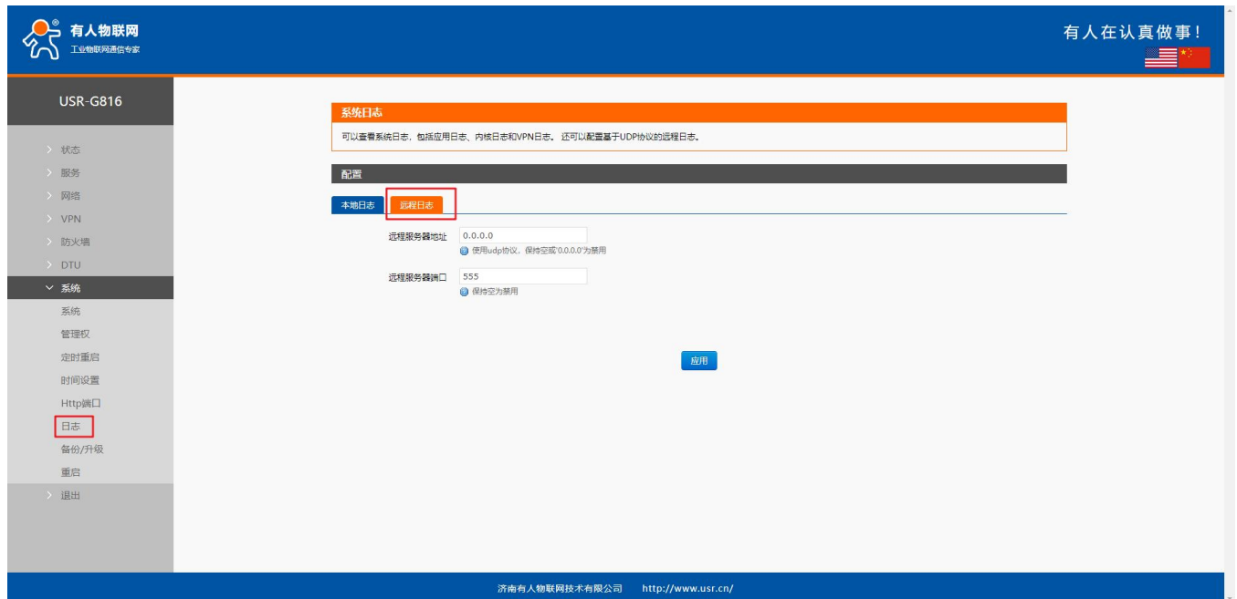
图 14 远程日志
