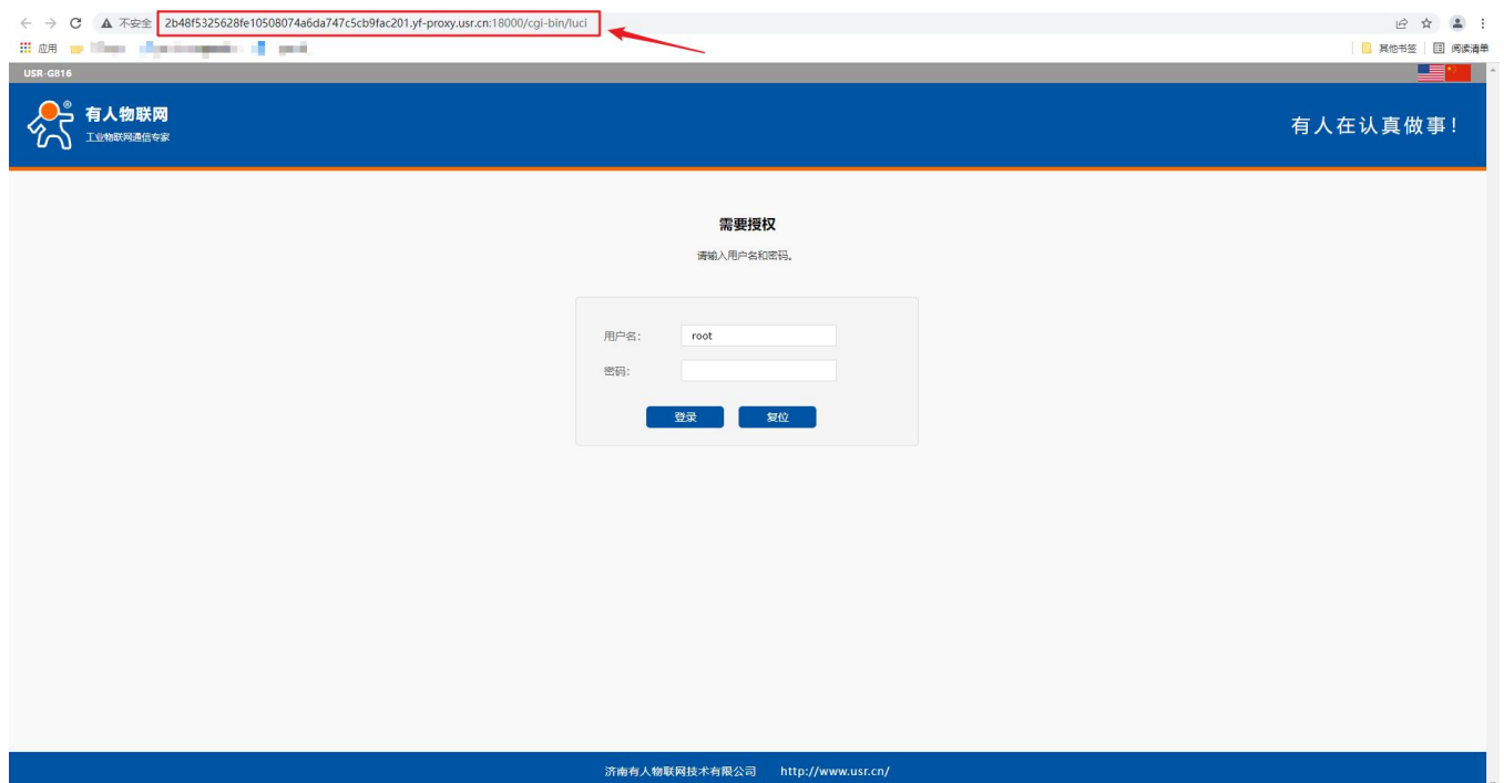
图 114 配置网页（二）
