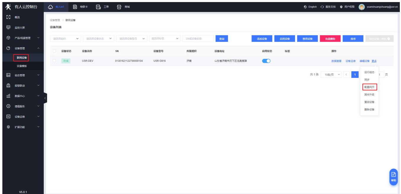
图 113 配置网页（一）
