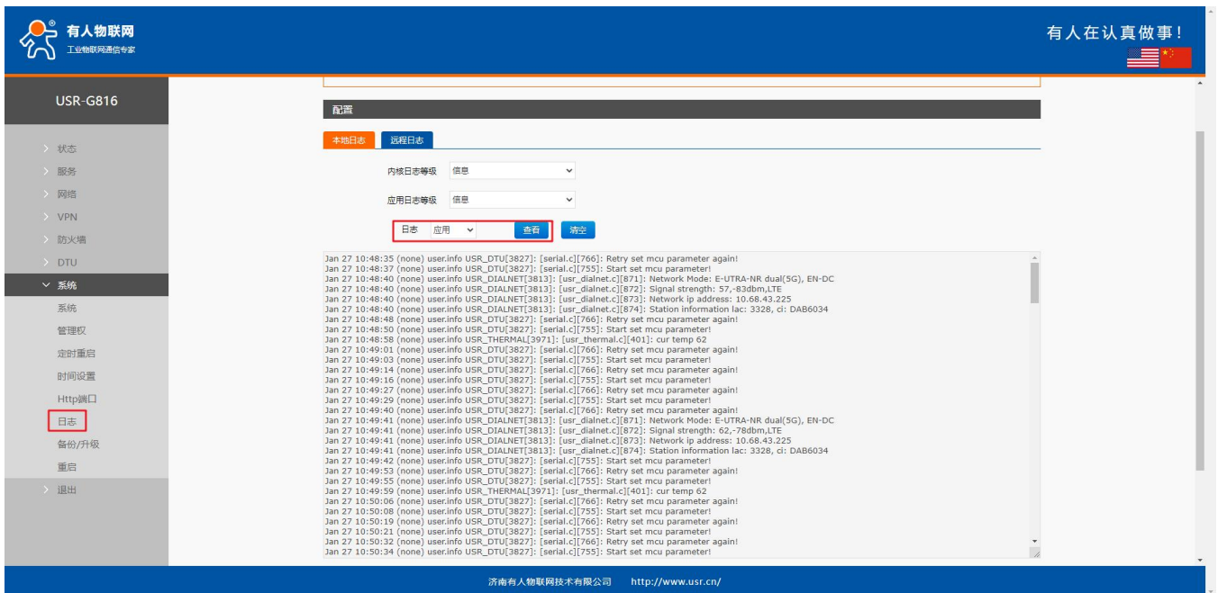
图 16 应用 log
