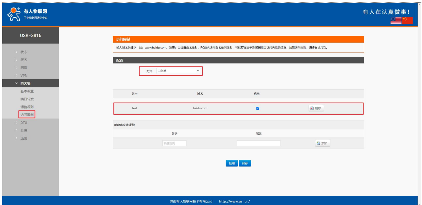
图 102 域名白名单
