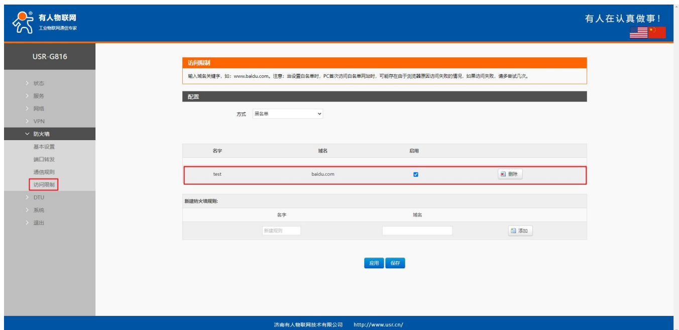
图 101 域名黑名单
