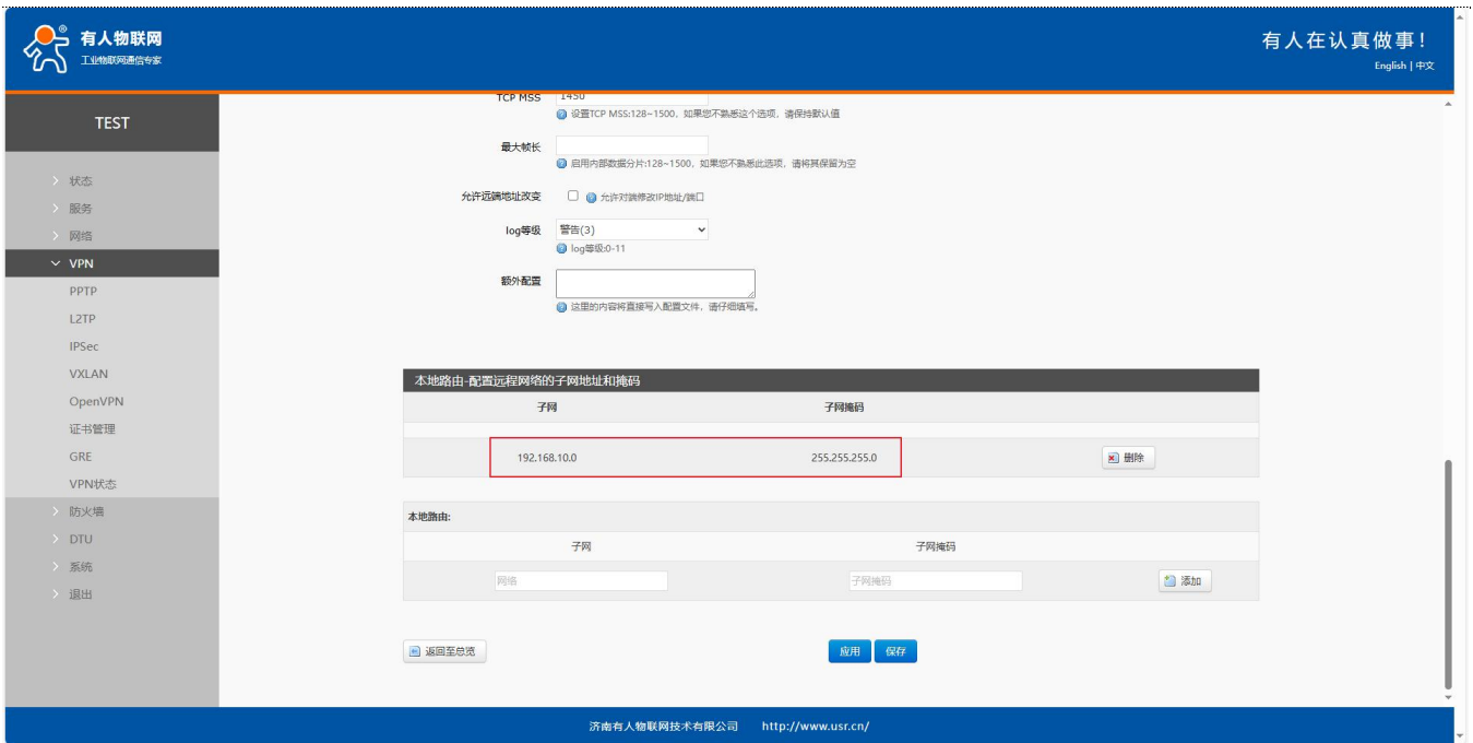
图 77 路由器 2 配置 2
