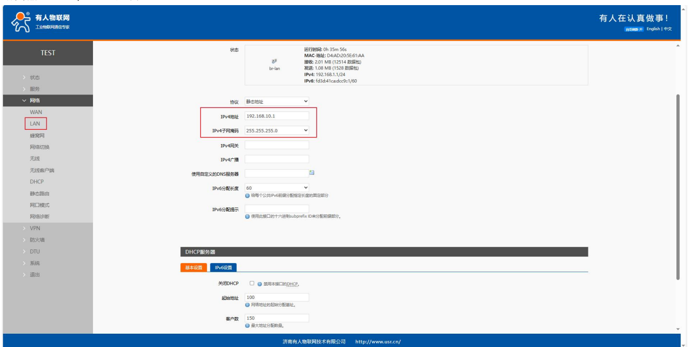
图 72 路由器 1 配置 1
