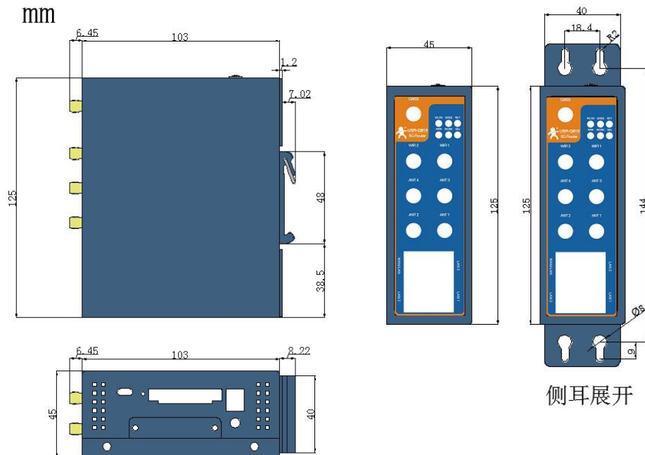
图 1 USR-G816 尺寸图
