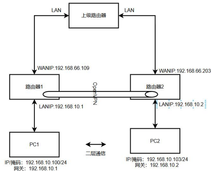
图 62 连接拓扑
