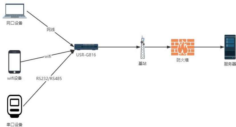
图 3 应用示意图
