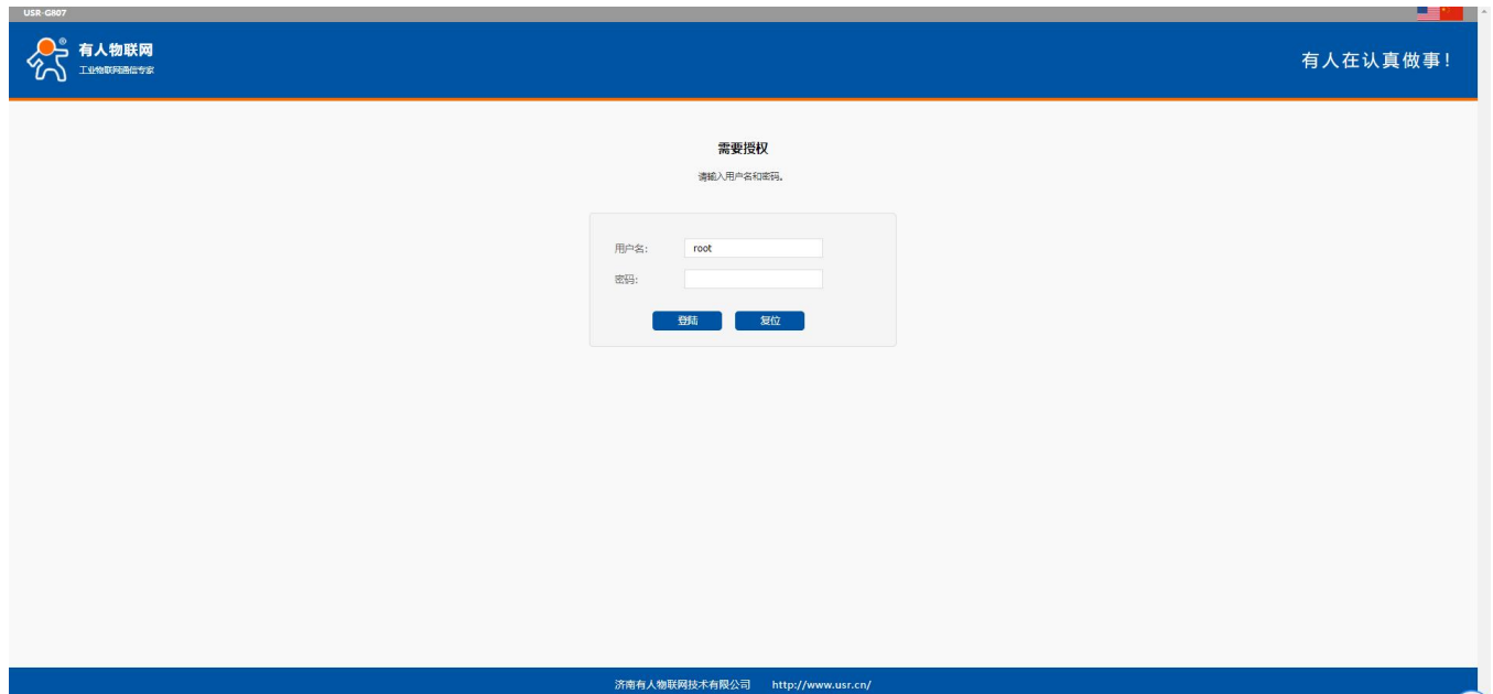
图 2 首页页面
