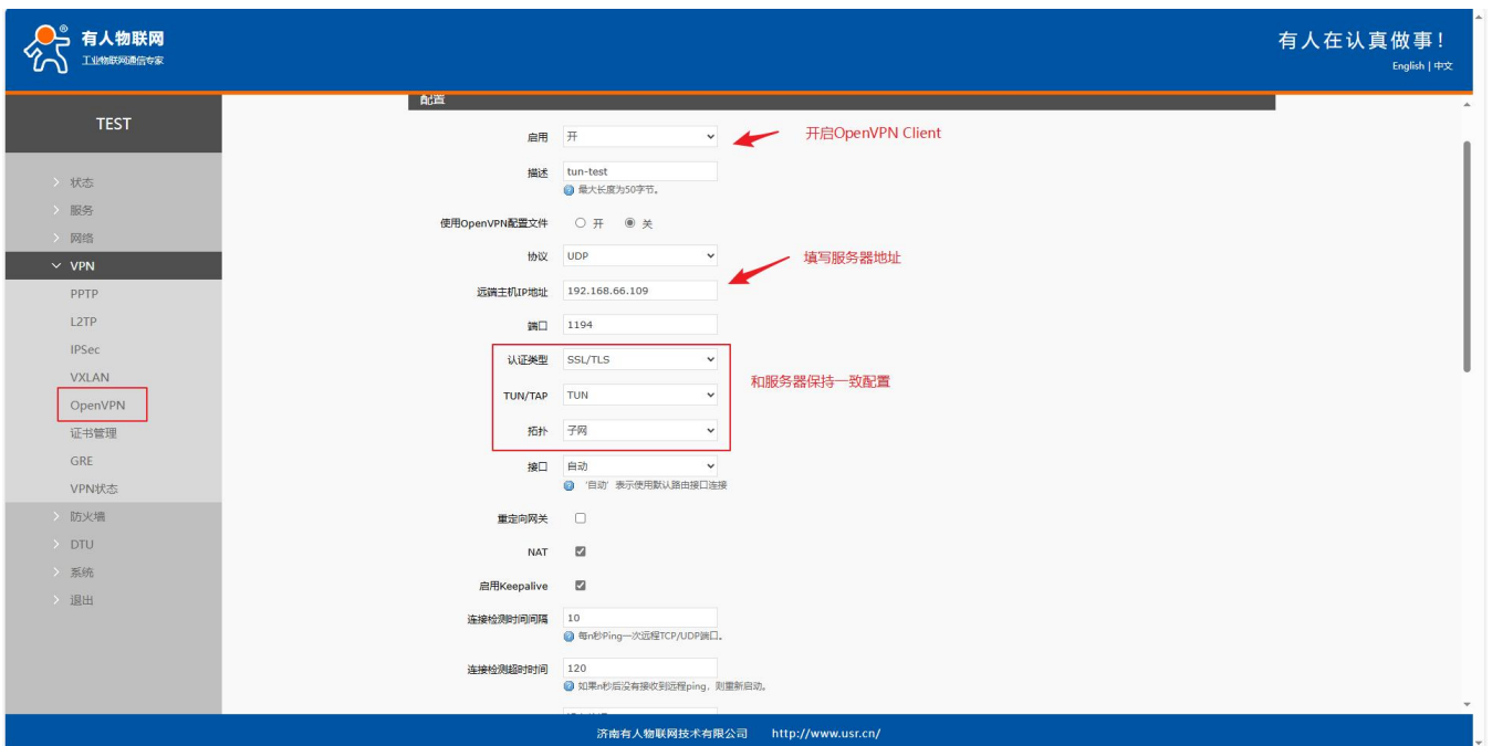
图 76 路由器 2 配置 1
