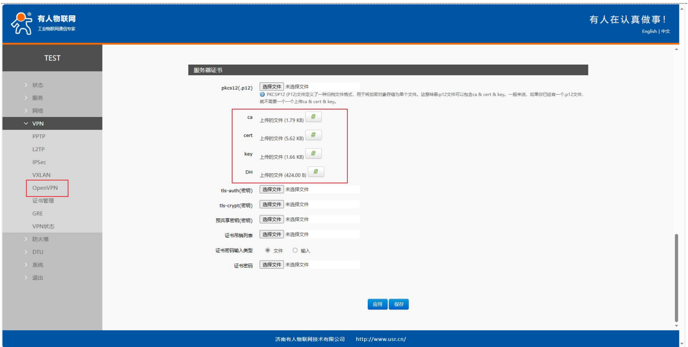
图 66 Openvpn 配置 3
