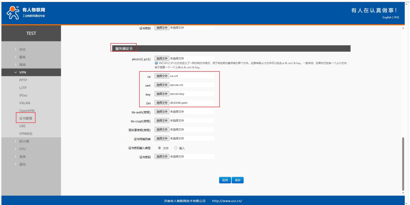
图 75 路由器 1 配置 4
