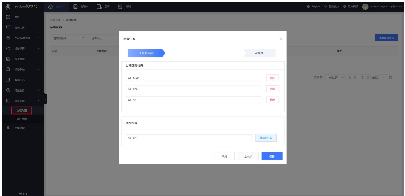
图 117 远程配置（三）
