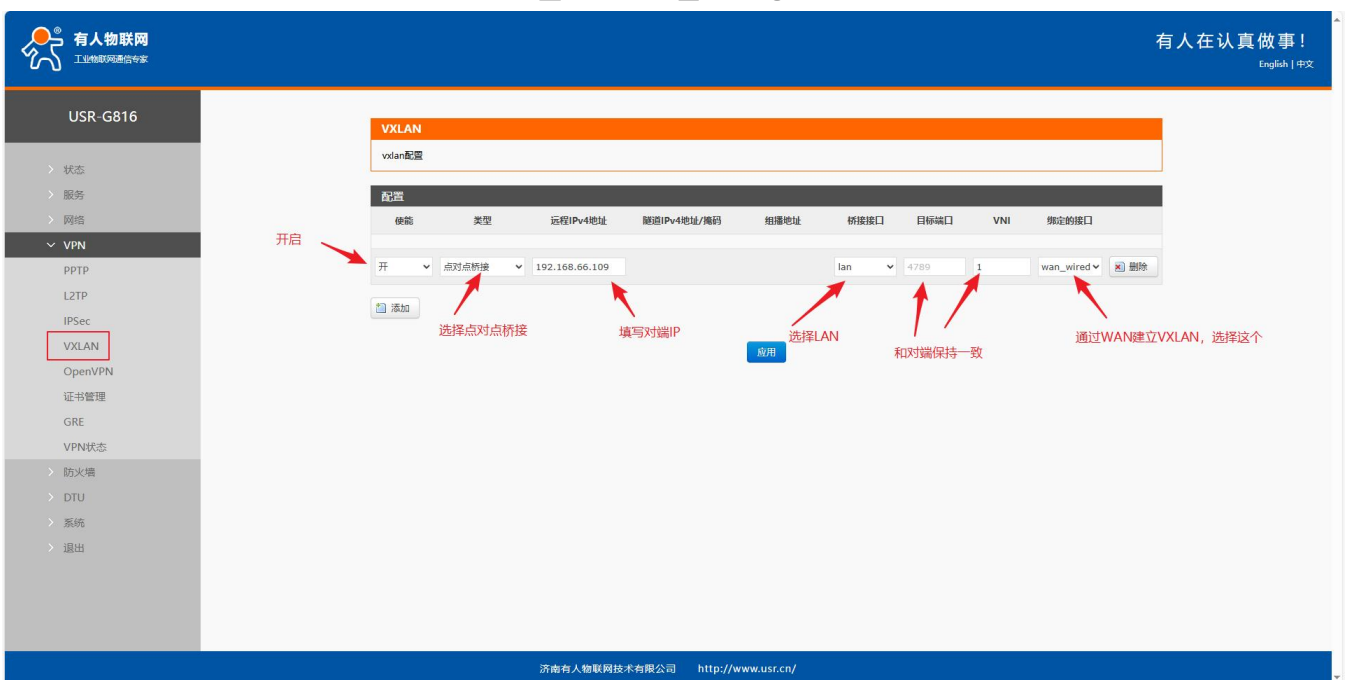
图 54 路由器 2 配置
