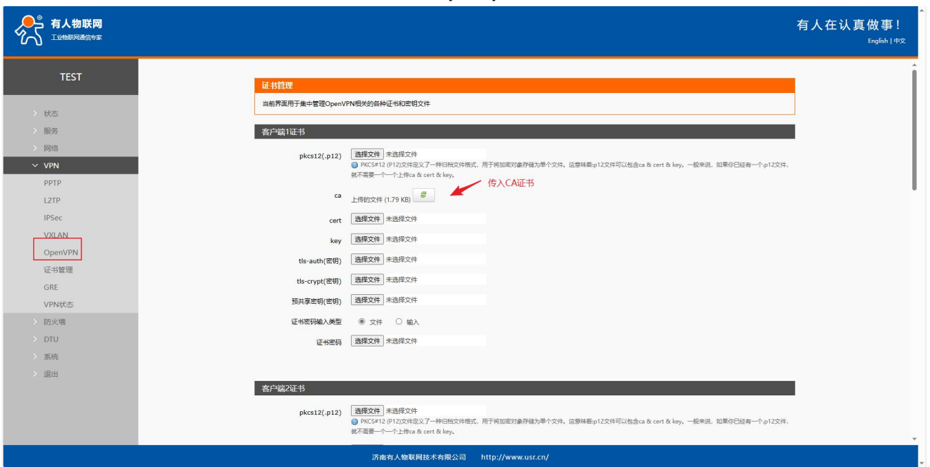
图 69 Openvpn 配置 2
