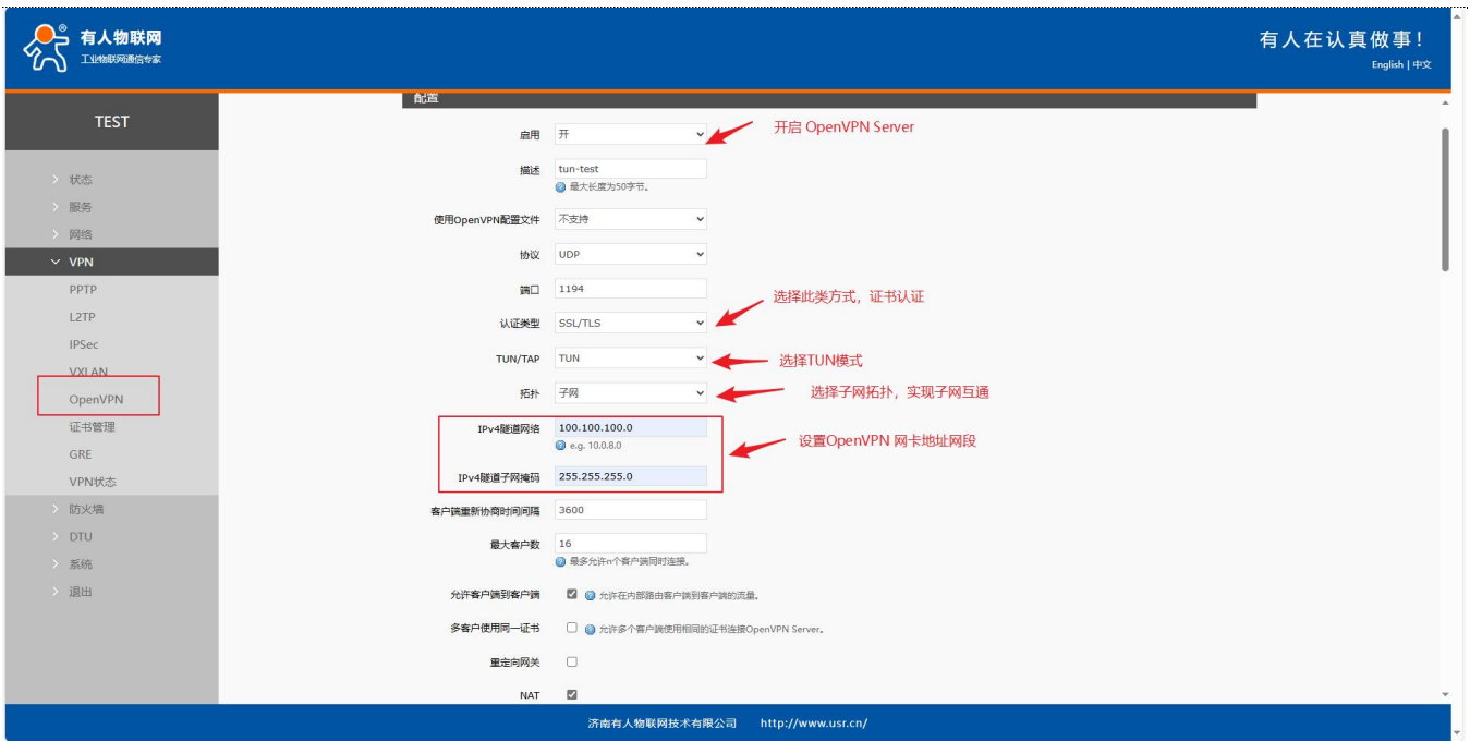
图 73 路由器 1 配置 2
