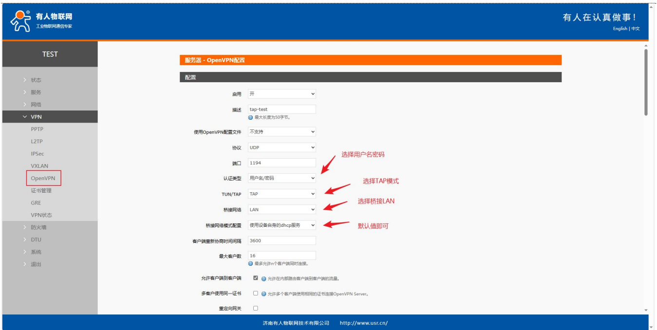
图 64 Openvpn 配置 1
