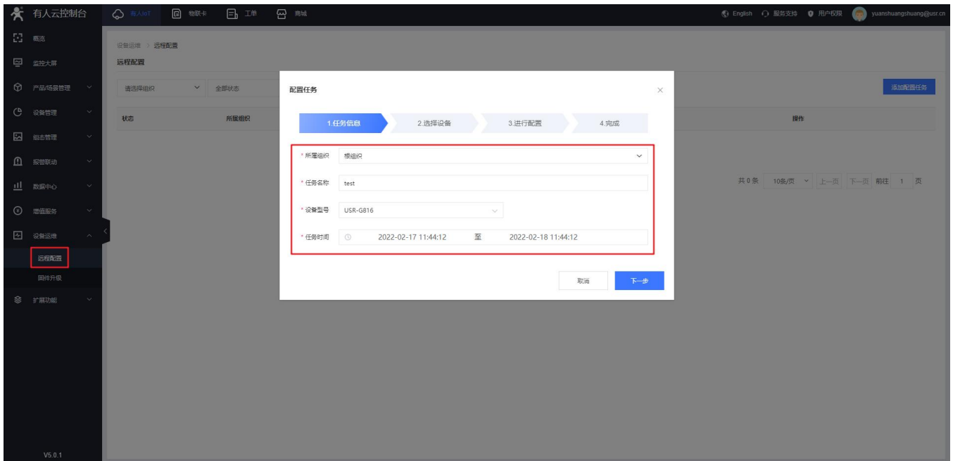
图 115 远程配置（一）
