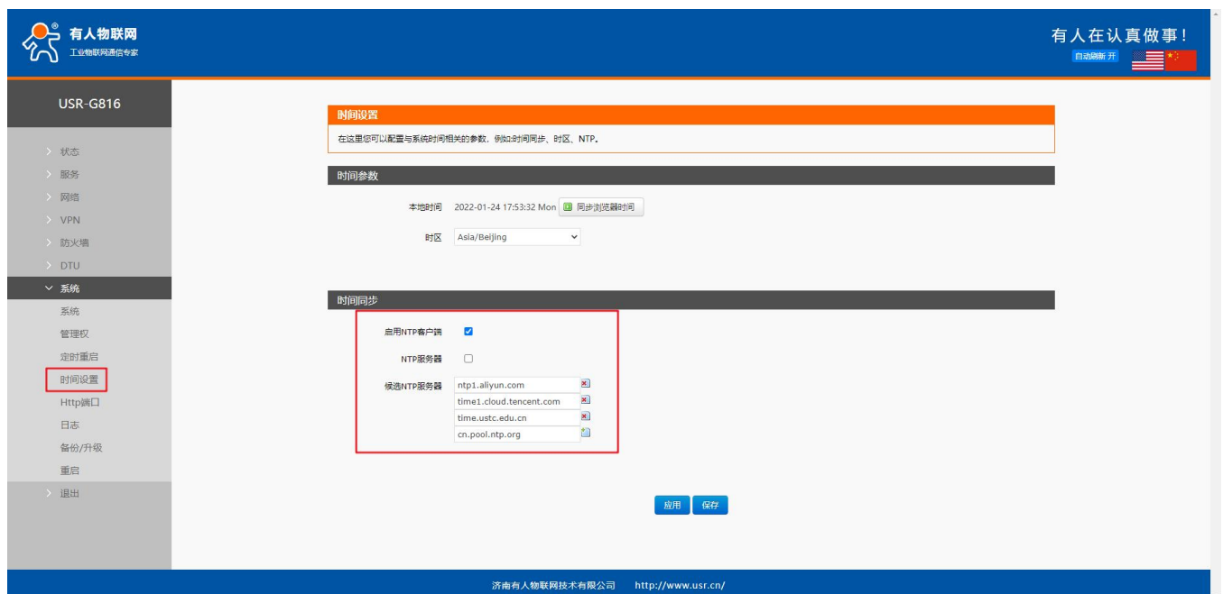
图 6 NTP 页面
