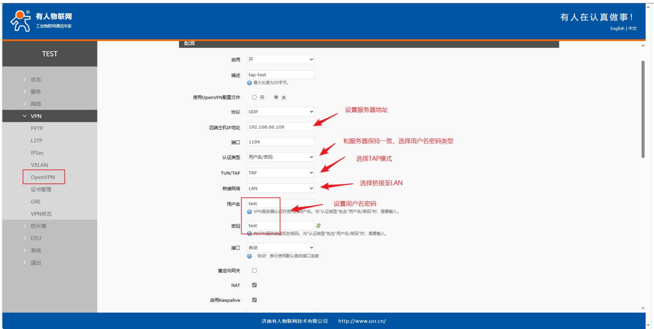
图 68 openvpn 配置 1
