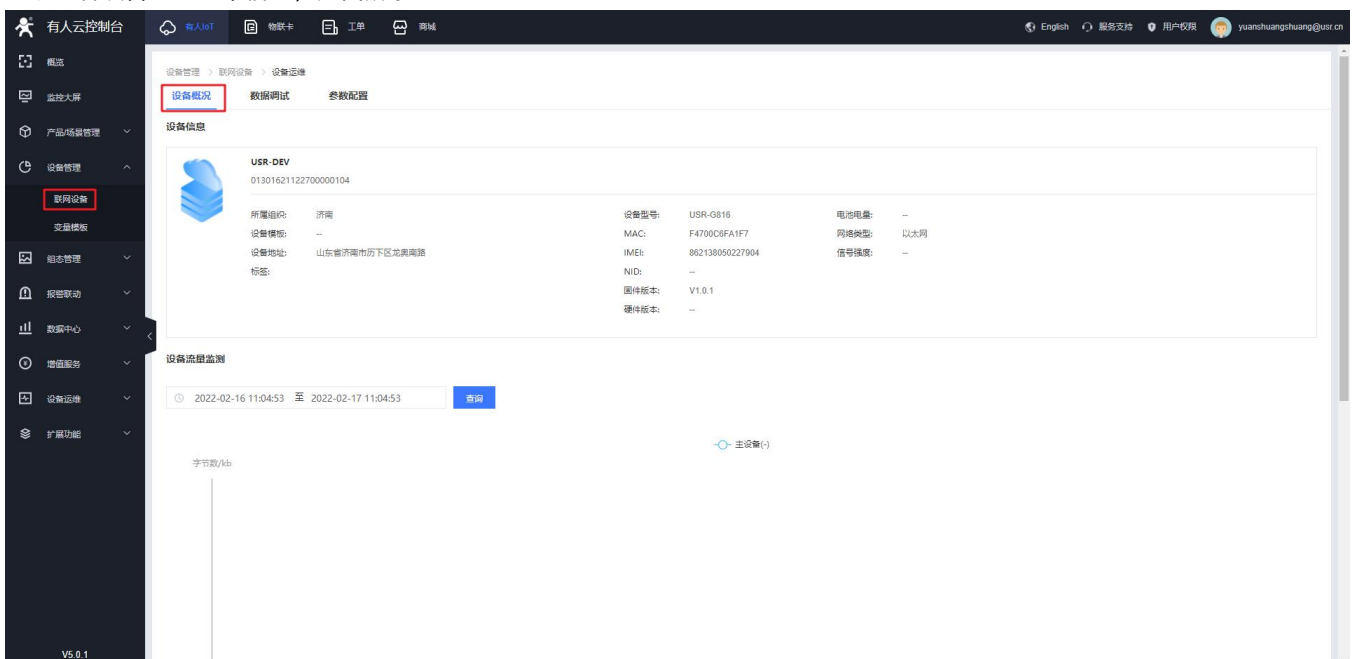
图 110 设备概况
