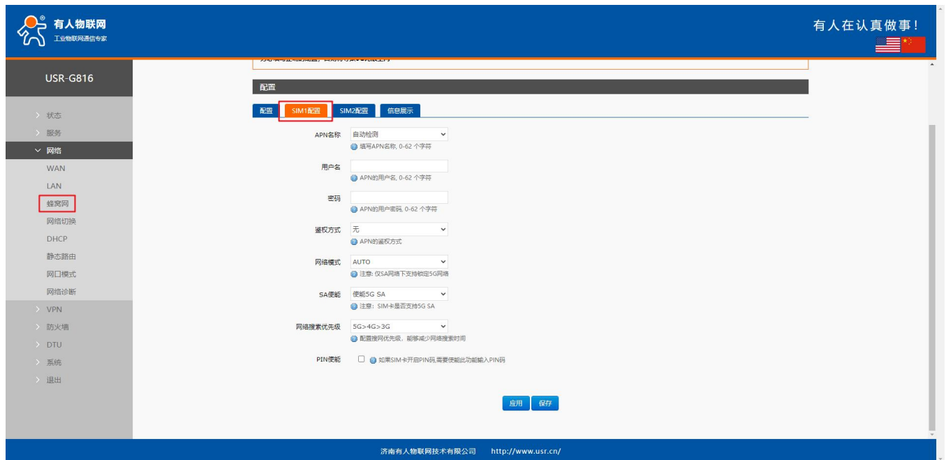
图 20 配置页面
