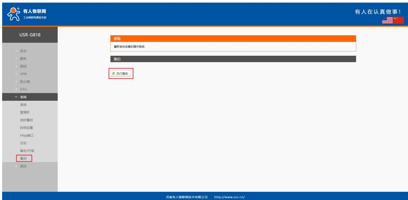
图 12 重启页面
