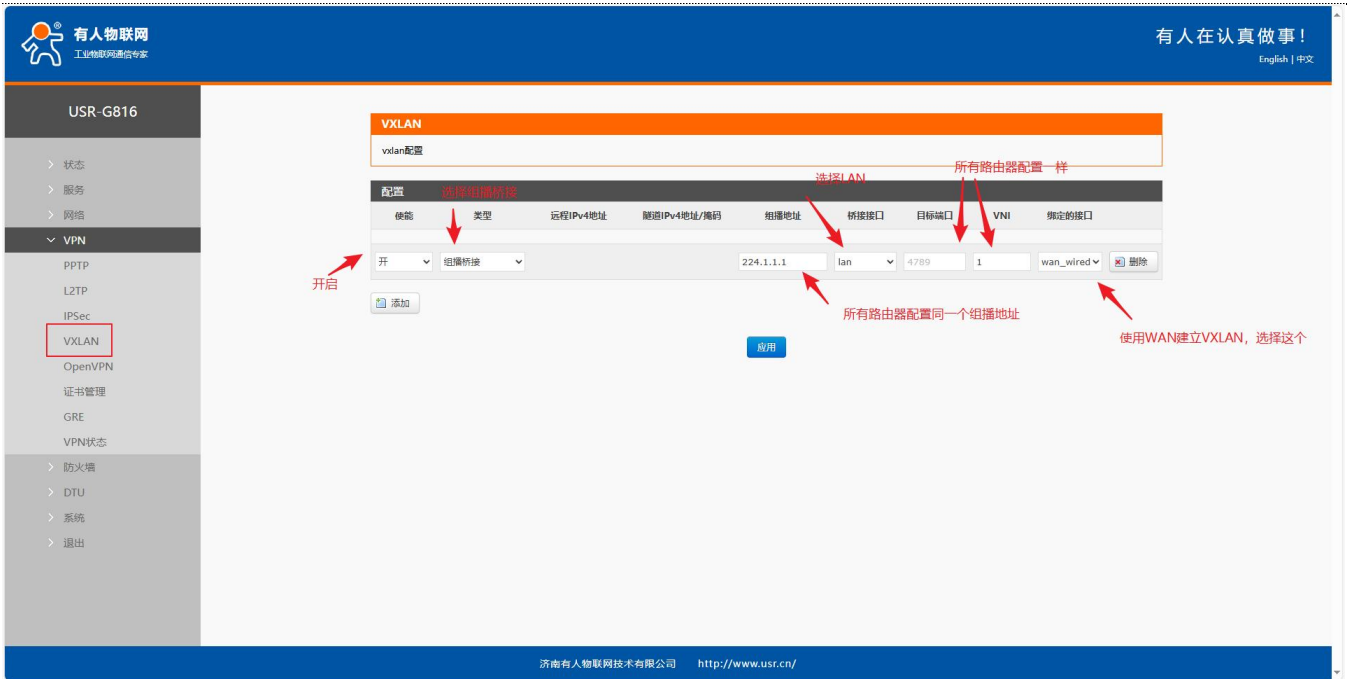
图 57 路由器 1 配置
