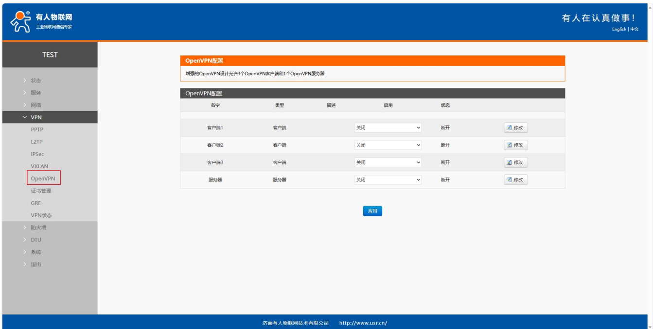
图 60 OpenVPN 页面
