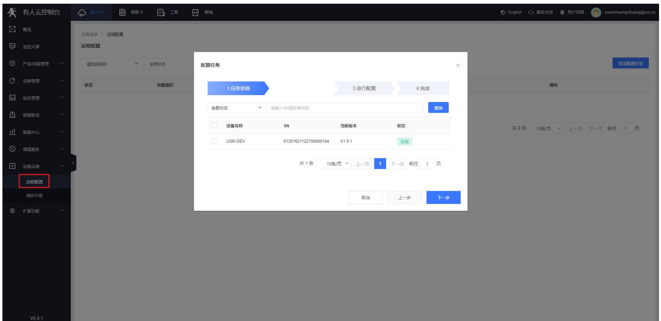
图 116 远程配置（二）
