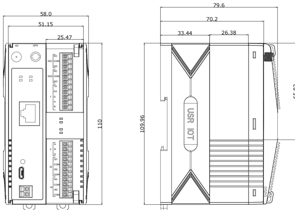
图 1. 尺寸结构图
