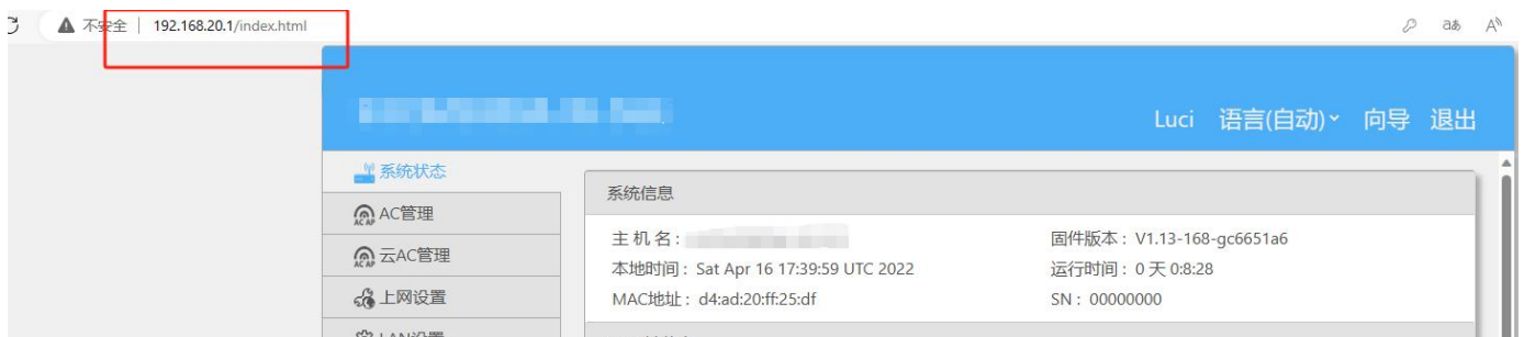
图 20 访问 WEB
