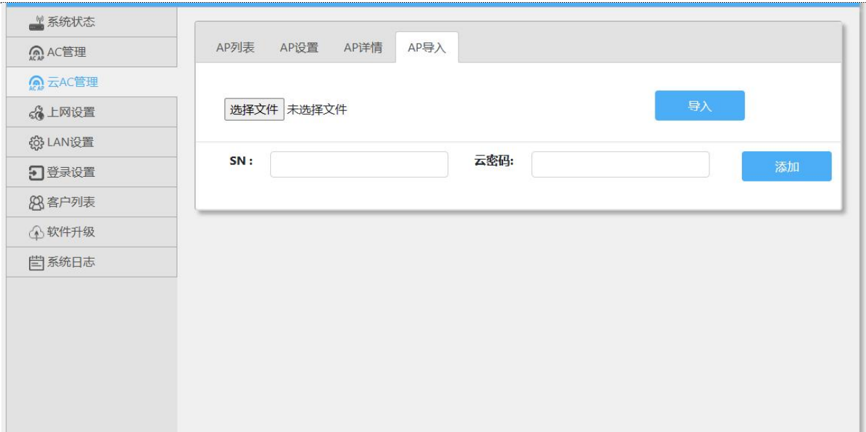
图 11 AP 导入
