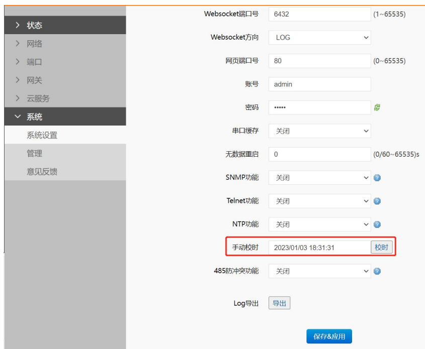
图 39. 校时设置
