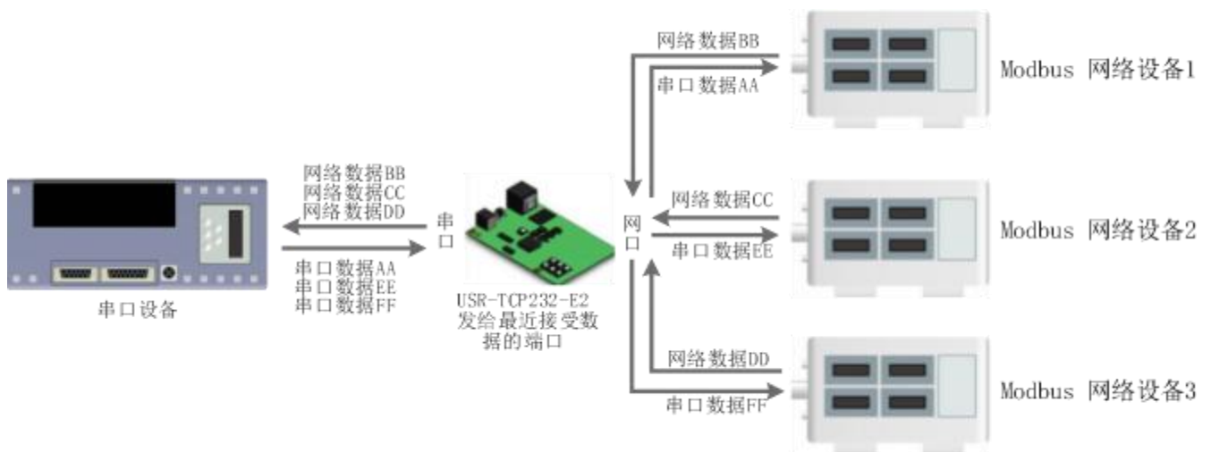
图 67 Modbus TCP
