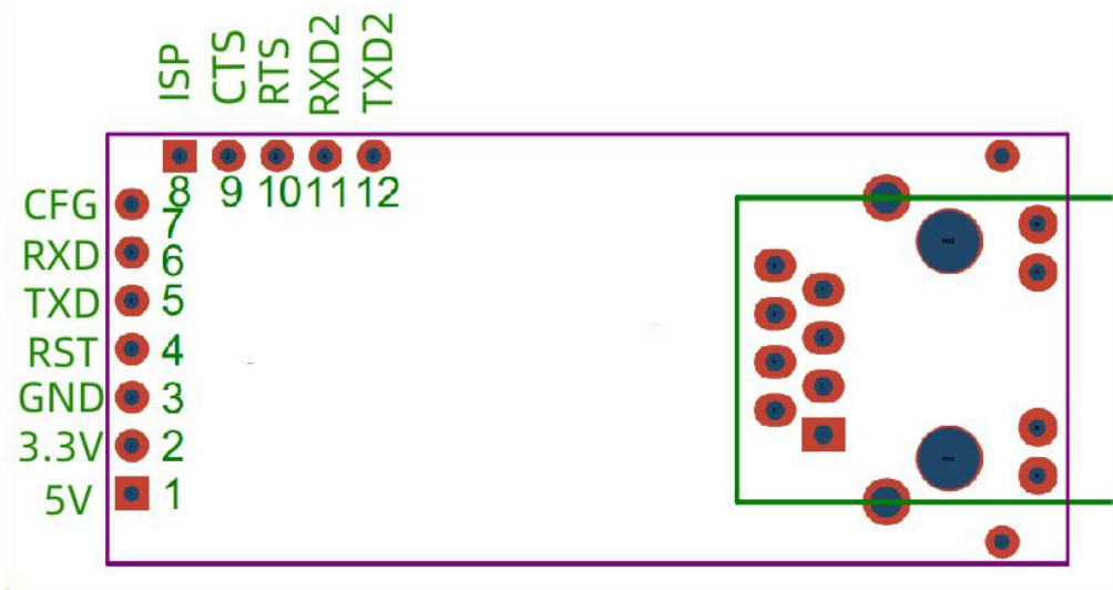
图 1. USR-TCP232-T1 模块接口定义 表 1 USR-TCP232-T1 模块管脚说明
