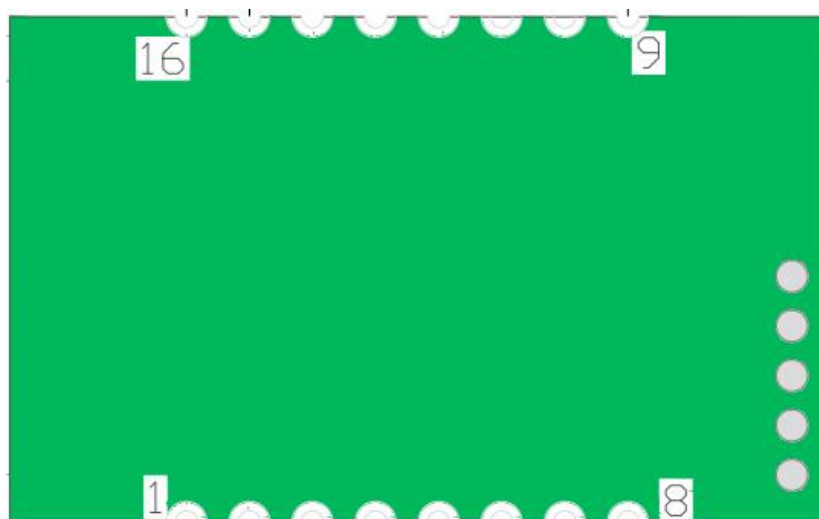
图 6. USR-TCP232-S2 模块接口定义
