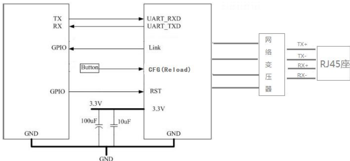
图 8. 硬件连接图
