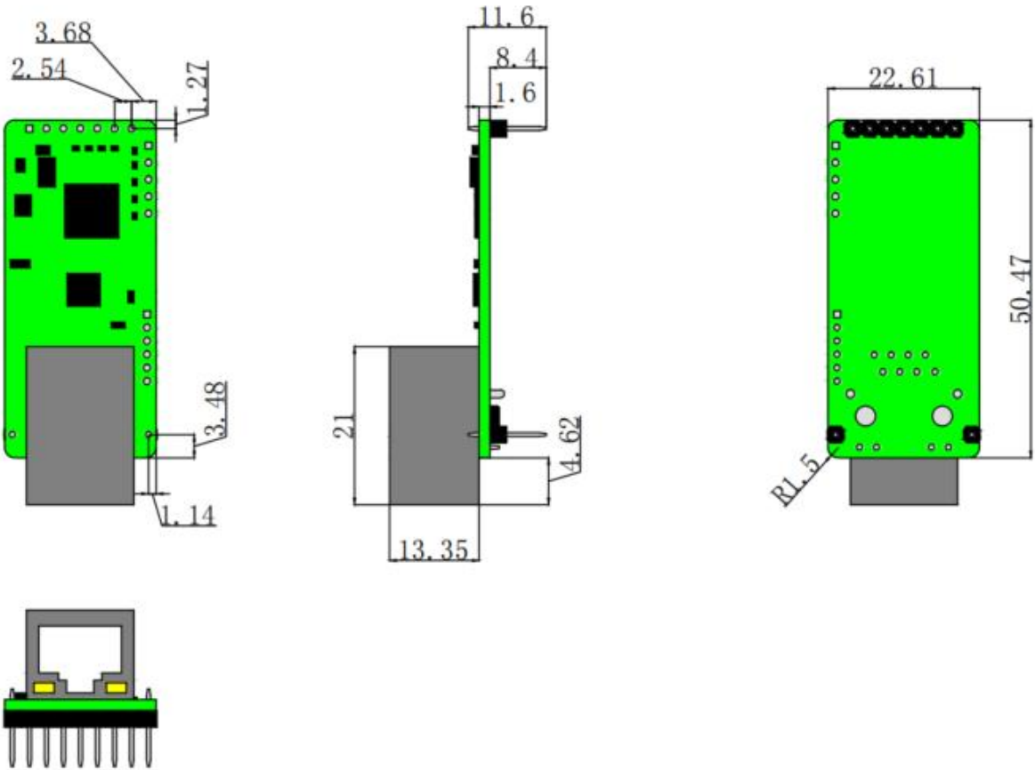
图 2. USR-TCP232-T1 尺寸图
