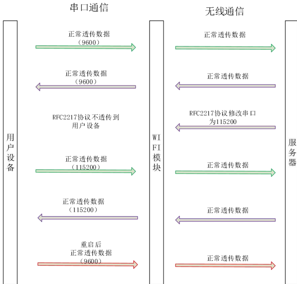
图 15 类 RFC2217 功能框图
