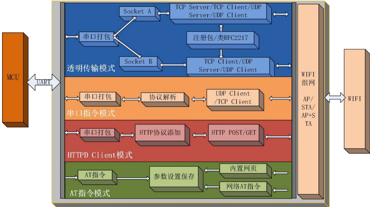
图 2 功能框图
