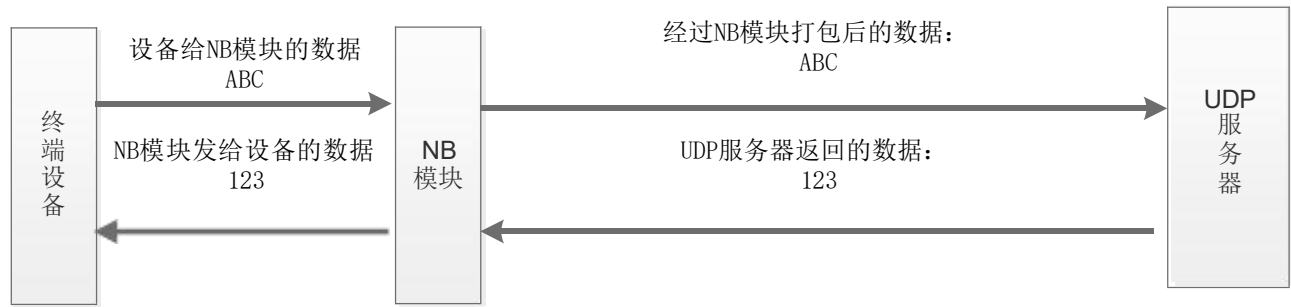
图 5 简单透传模式示意图
