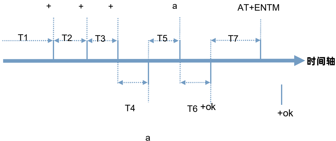
图 2 进入串口 AT 命令模式时序
