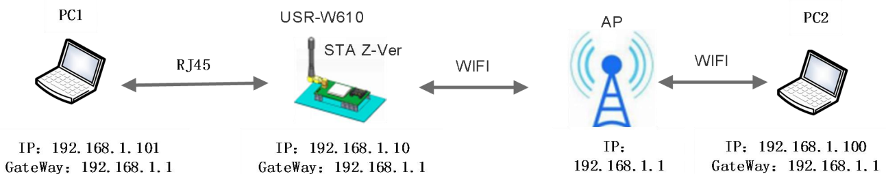
图 18 有线加无线组网应用（桥接）
