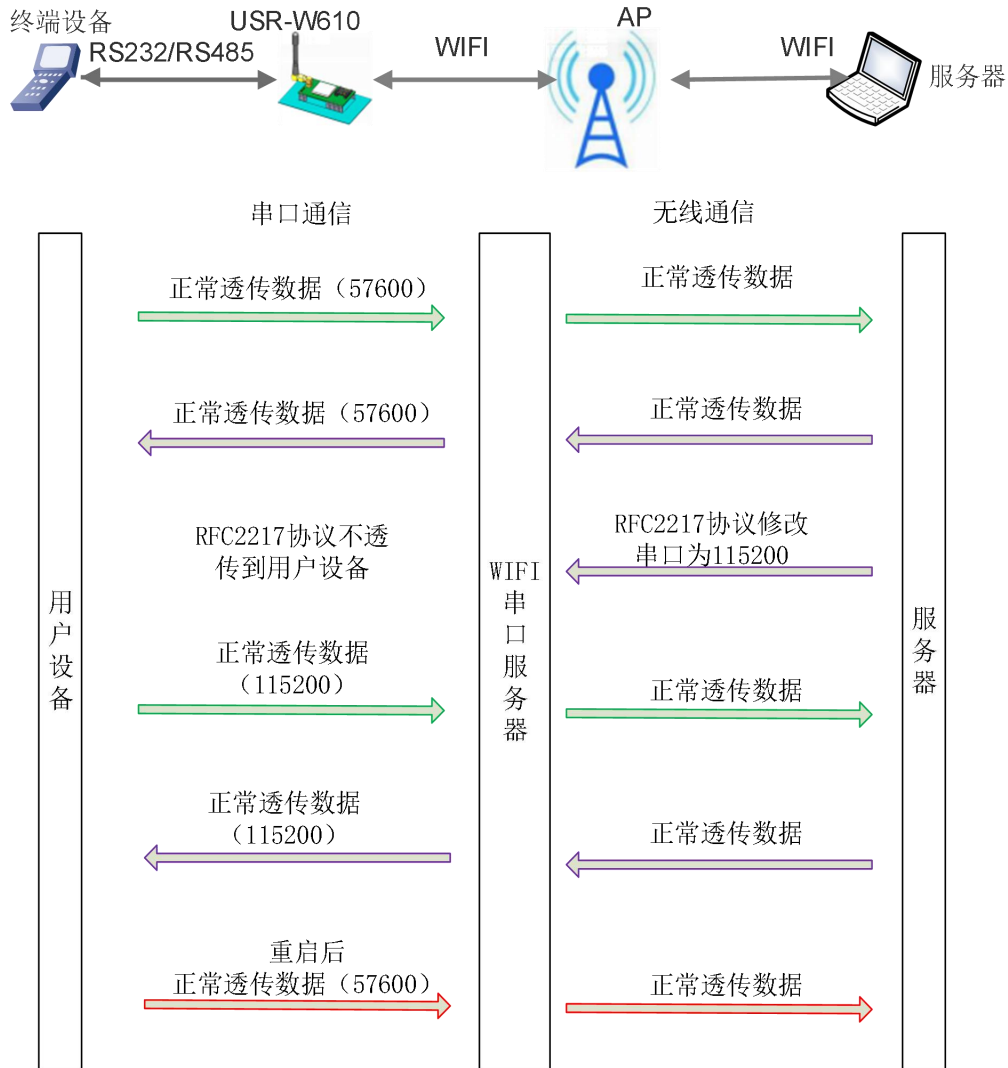
图 29 类 RFC2217 自动波特率框图
