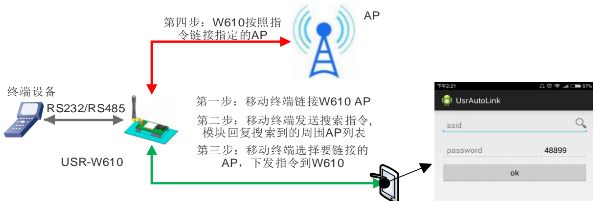
图 31 usr-link 框图
