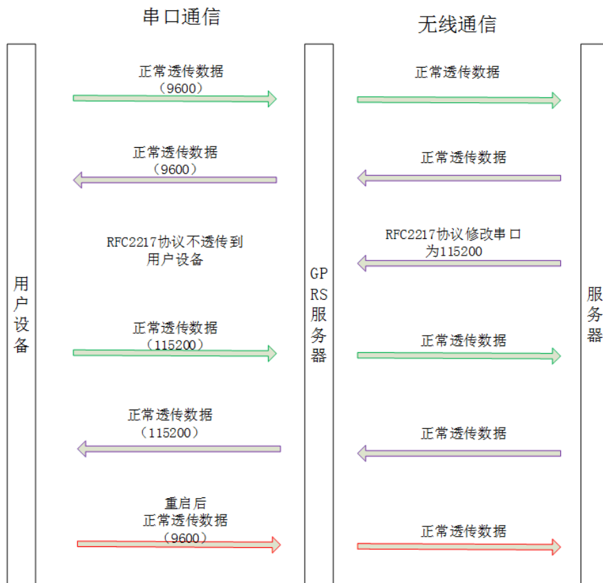
图 13 类 RFC2217 功能逻辑示意图
