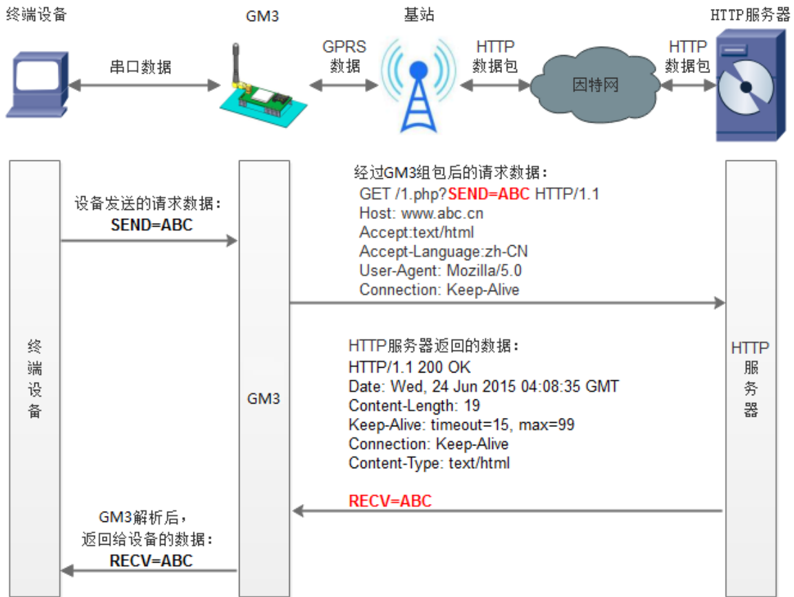
图 5 HTTPD 模式
