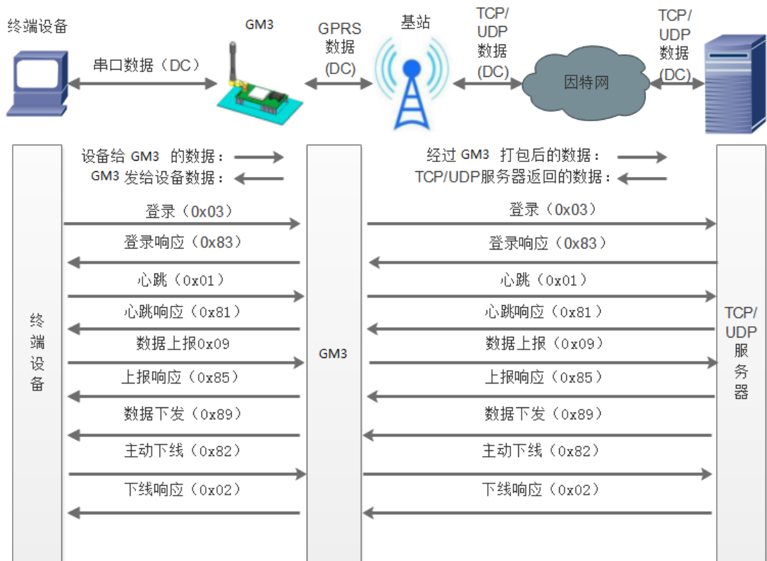
图 10 UDC 模式
