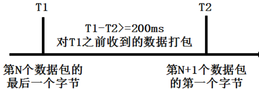
图 12 成帧机制示意图
