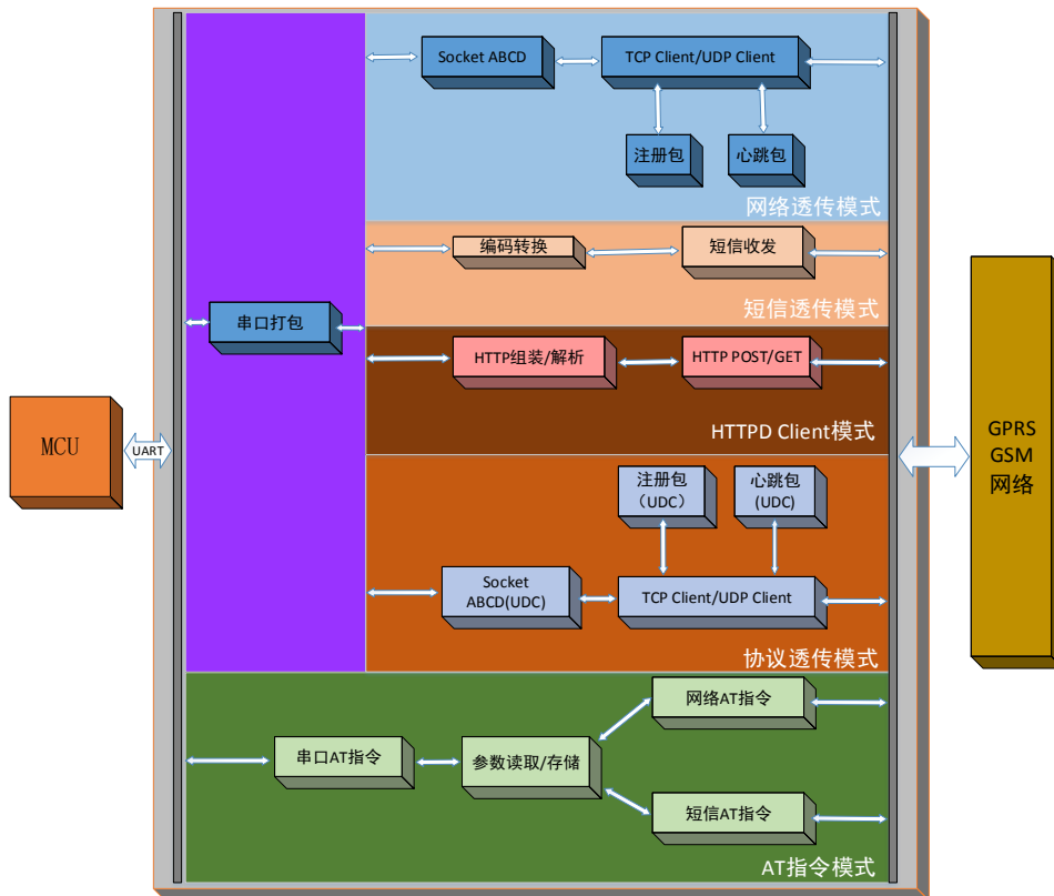
图 2 功能框图
