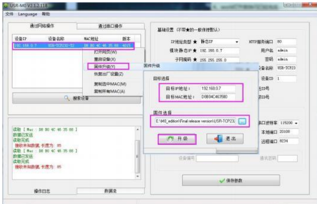
图 5. 选择固件
