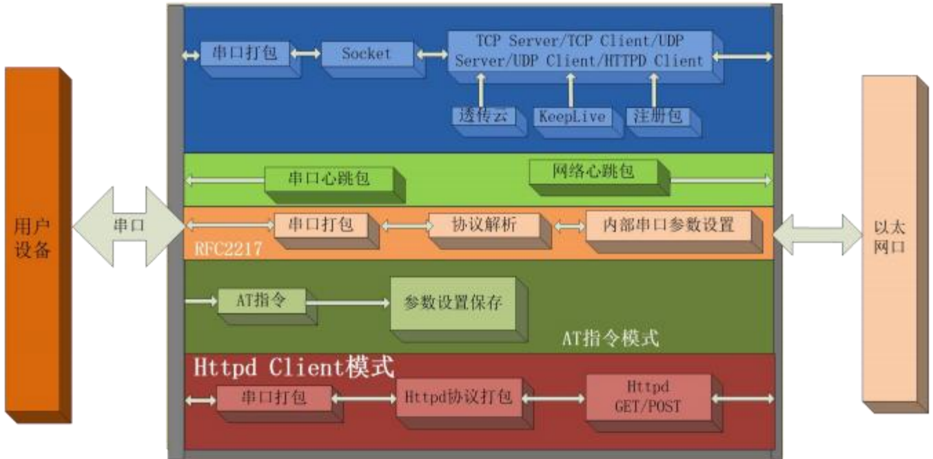
图 1. T2 功能框图
